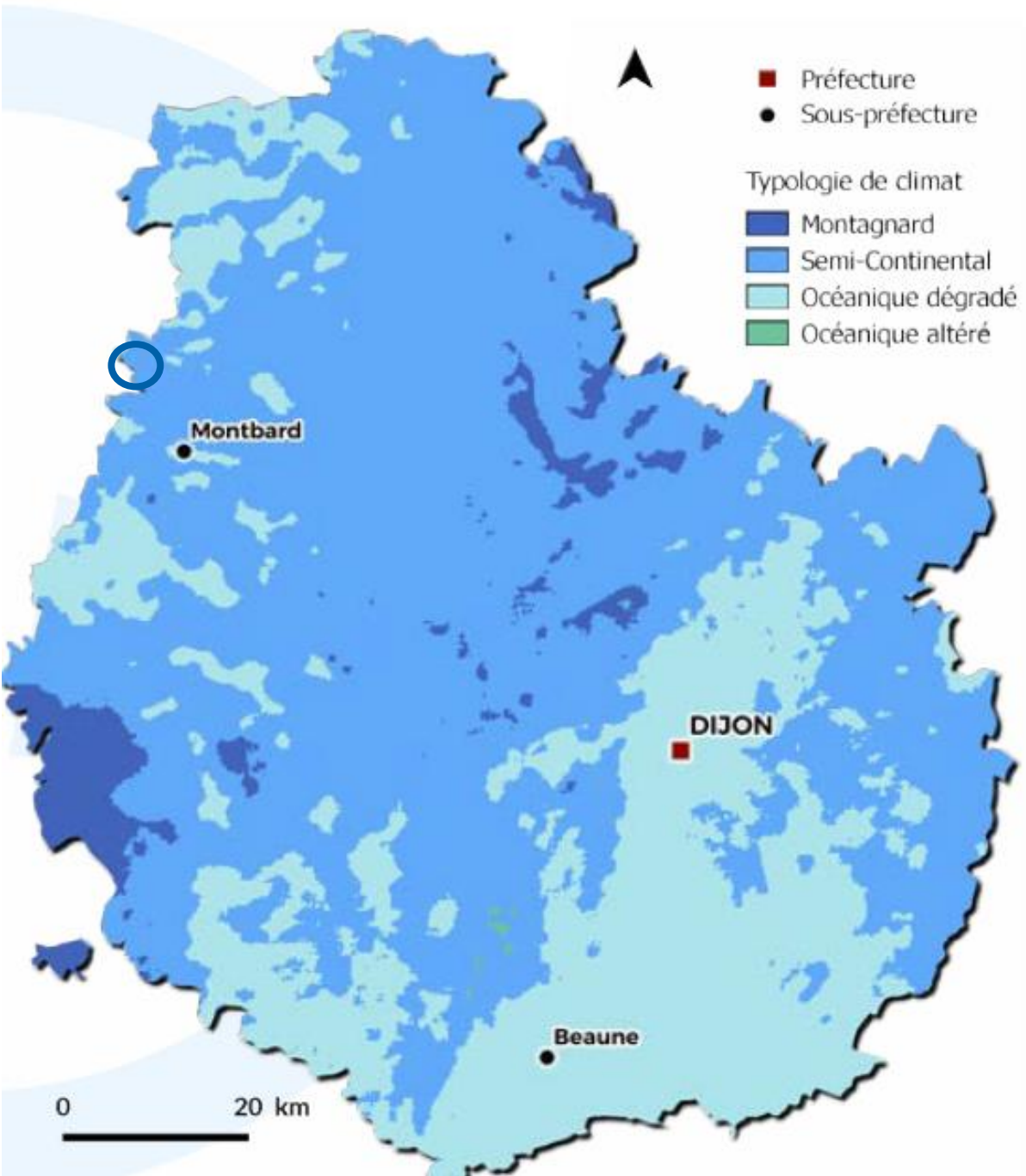
Carte 4 : Climats de de la Côte d'Or – Cercle bleu : Périmètre d'étude de dangers (source : DDRM de la Côte d'Or, 2019)
